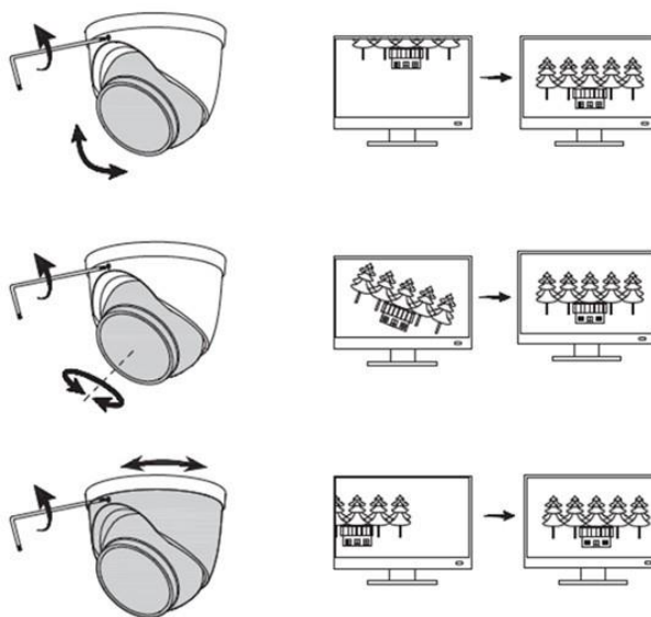
Figure 3-6. Réglage de l'angle de l'objectif
