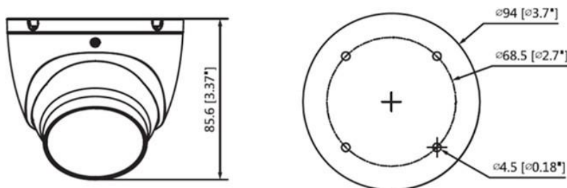
Рис. 3-1 Размеры (единицы измерения: мм [дюймы])
