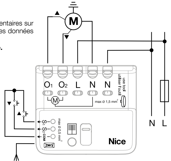
Figure 2 : Schéma de câblage du BiDi-MiniShutter
