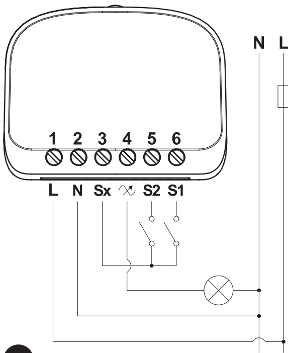
2 Installation à 3 fils (avec Neutre)
